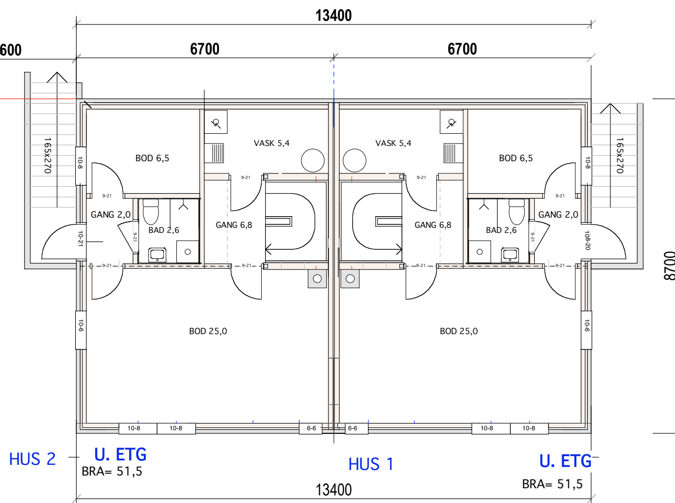
E.1-4 Plan u.etg
