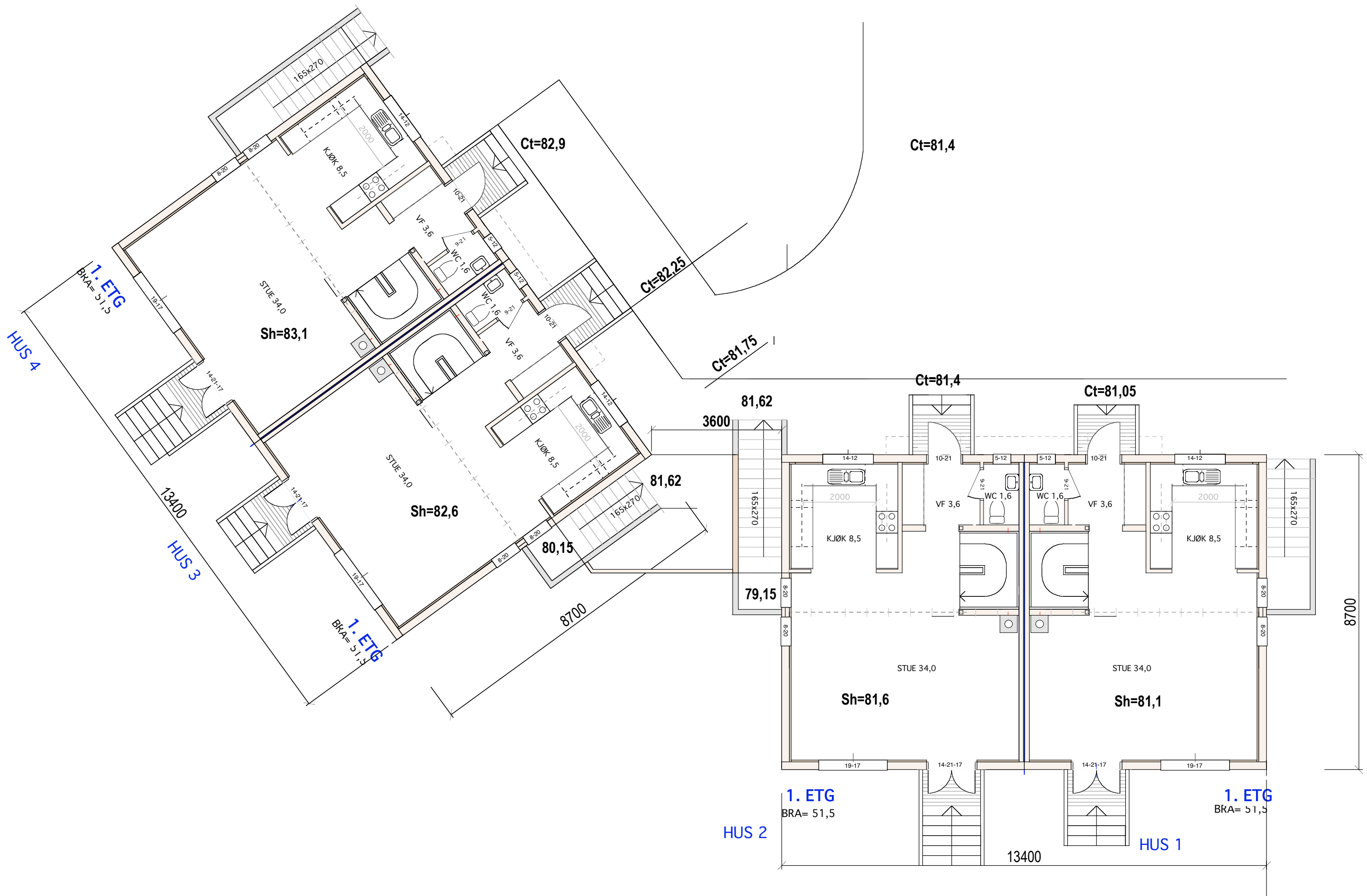
E.1-3 Plan 1.etg
